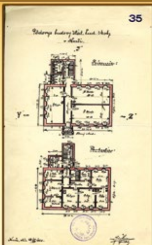
Obr. č. 7 Pôdorys budovy školy z roku 1928
